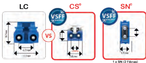
Comparacion de tamaño entre conectores LC, CS® y SN®
