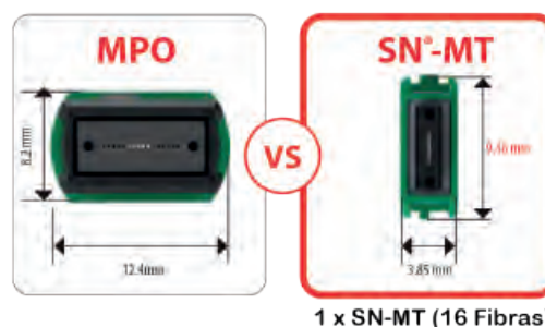
Comparacion de tamaño entre conectores MPO y SN-MT
