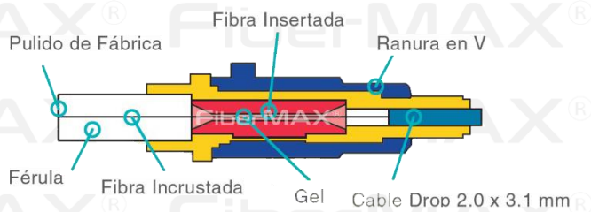
Detalle constructivo
