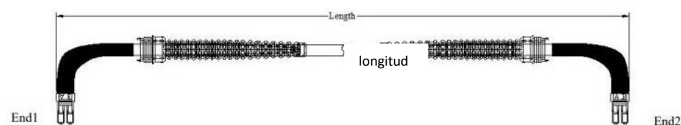
Patchcord dúplex NSN bota 90°
