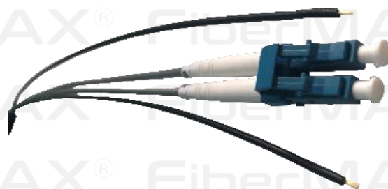
Terminación CPRI-LC Dúplex
