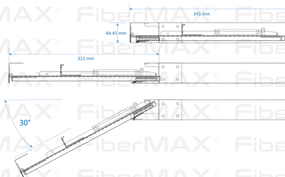
Vista Lateral
