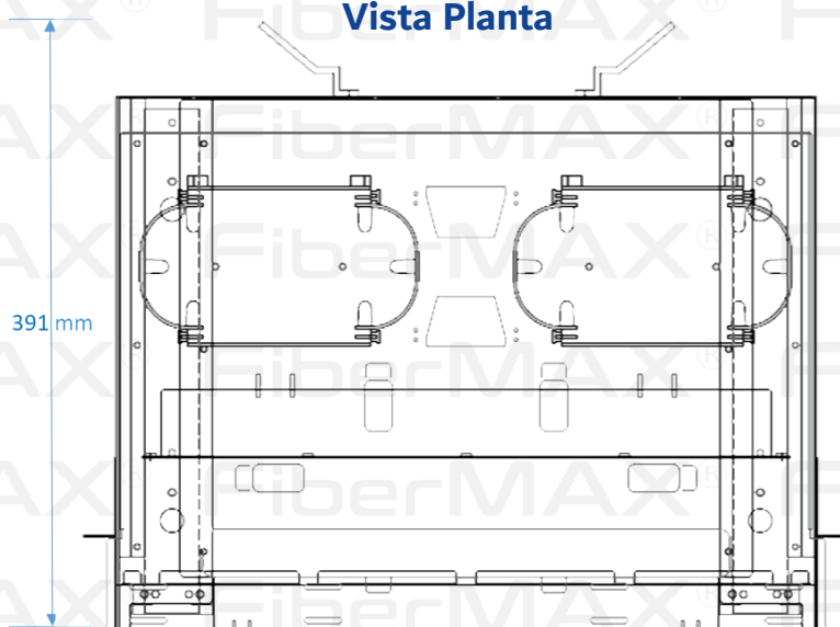
Vista Planta
